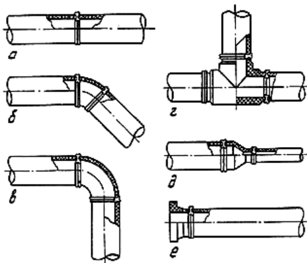
Рис. 4. Сварные стыковые соединения труб и соединительных деталей из ПНД: а - трубы с трубой; б, в - труб с угольниками соответственно 45° и 90°; г - труб с тройником; д - труб с переходом; е - трубы с втулкой под фланец
