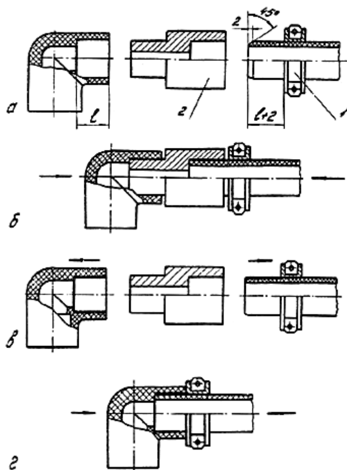
Рис. 9. Последовательность процесса контактной сварки впаструб труб и соединительных деталей из ПВД: а - центровка, закрепление в зажимах сварочного устройства концов свариваемых труб и деталей и установка ограничительного хомута 1; б - установка дорна нагретого инструмента 2 в раструбе и гладкого конца трубы в гильзе; в - нагрев (оплавление) свариваемых концов, одновременно снятие их с дорна и гильзы; г - соединение концов с выдержкой до затвердевания сплавленного материала
