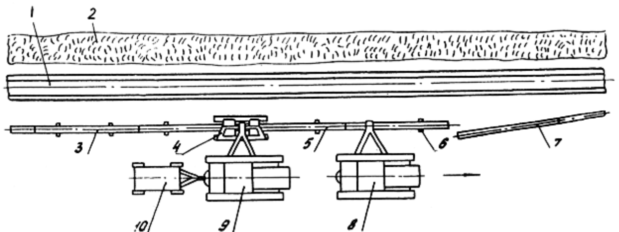
Рис. 14. Схема сварки трубопровода в непрерывную нитку с использованием одного центратора и грузоподъемной техники:
