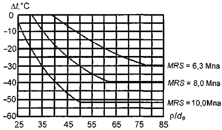
Рисунок 4 - Максимально припустимий негативний температурний перепад у залежності від відношення радіуса пружного вигину до зовнішнього діаметра газопроводу при температурі експлуатації 0°C и робочому тиску 0,3 МПа для SDR 11 і різних MRS
