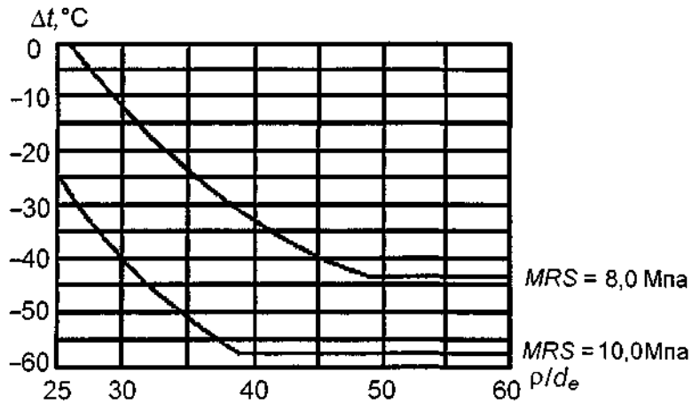
Рисунок 5 - Максимально припустимий негативний температурний перепад у залежності від відношення радіуса пружного вигину до зовнішнього діаметра газопроводу при температурі експлуатації 0°C и робочому тиску 0,6 МПа для SD.R 11 і різних MRS
